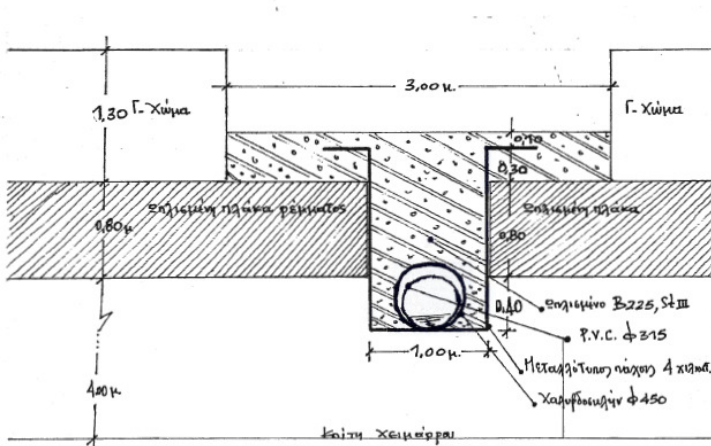
Τομή Β - Β
